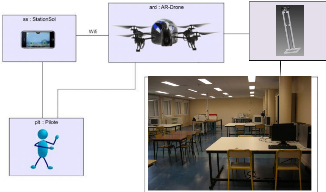
ibd[block] SystemeAR-Drone [Diagramme de contexte du systeme]
