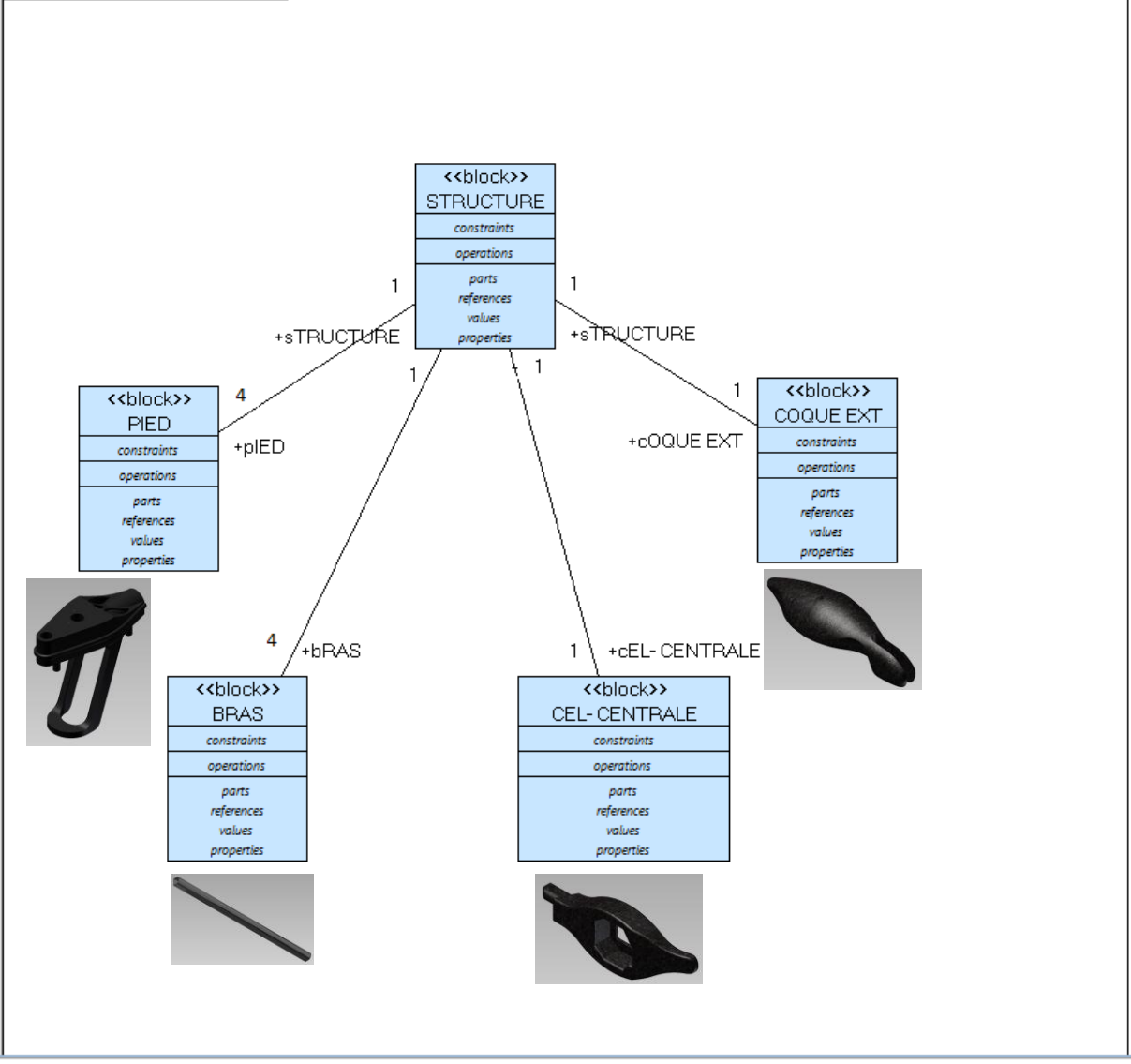
Diagramme BDD conforme à la représentation SYSML
